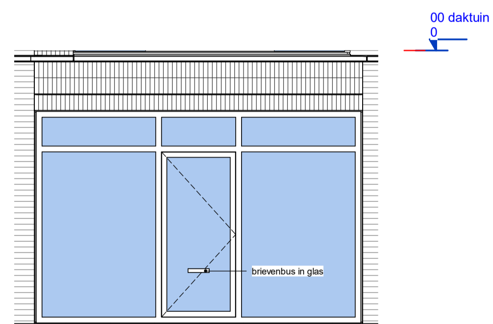
plint unit 7 schaal 1 : 50
