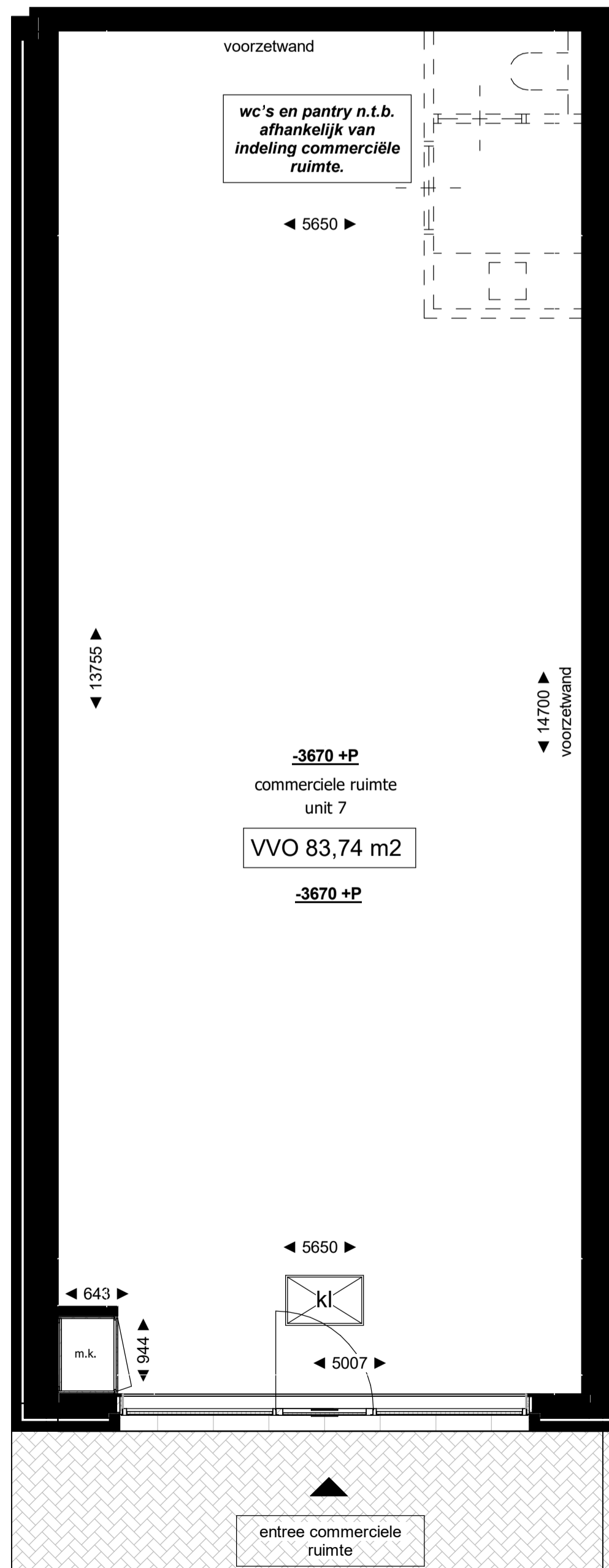
kadeniveau - unit 7 schaal 1 : 50
