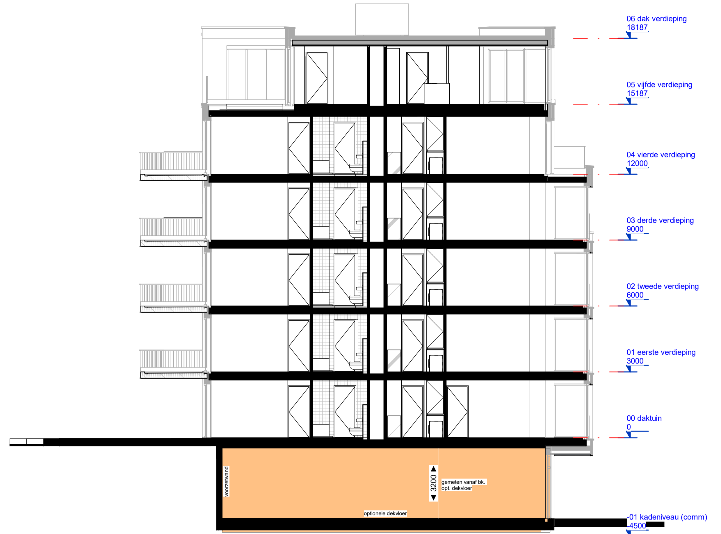
doorsnede - unit 7 schaal 1 : 100
